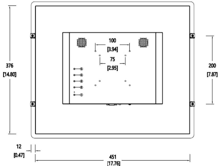
Abmessungen Ausbruch
