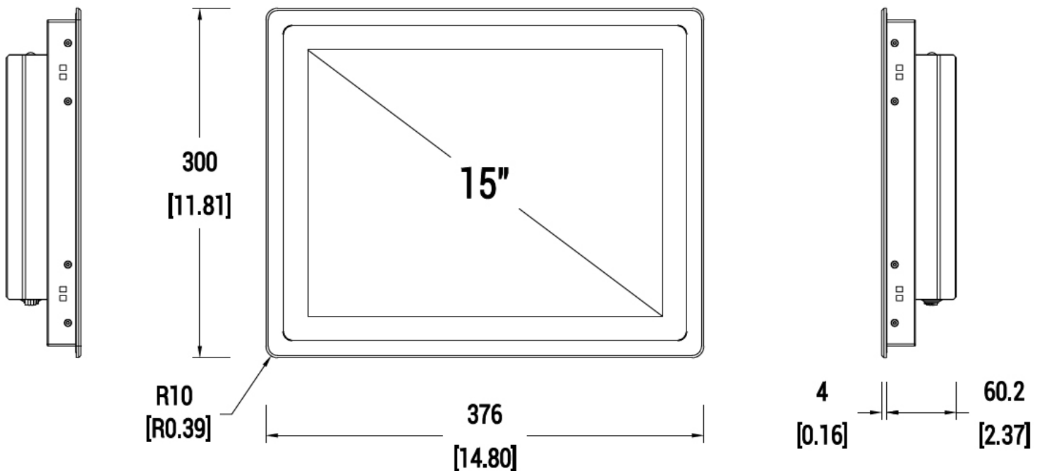
Frontansicht
